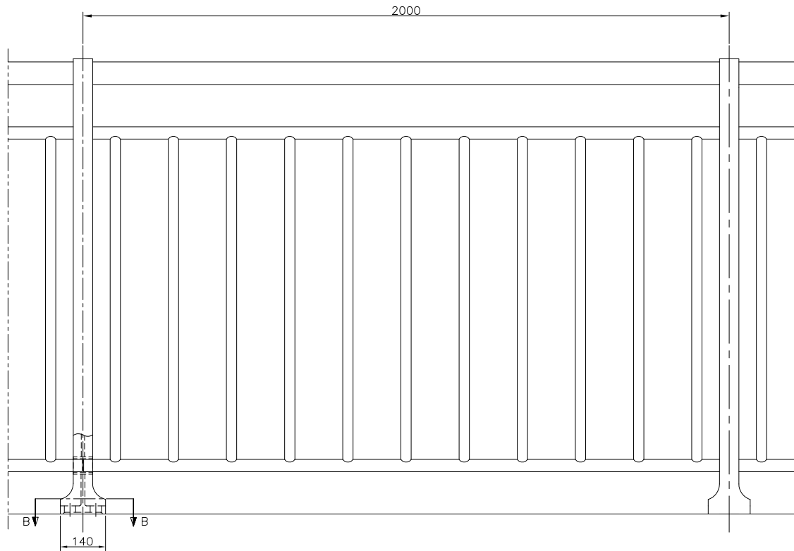
정면 상세도 S : 1/6
