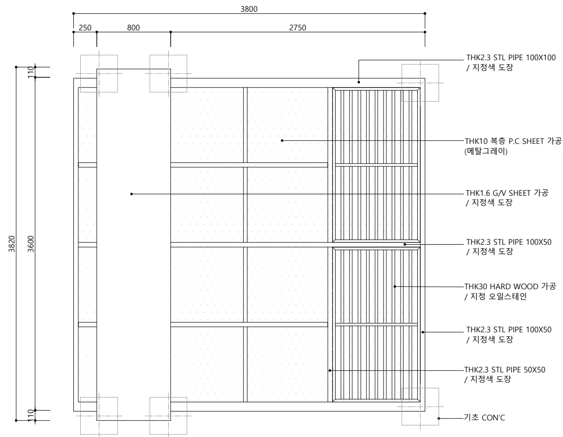
1 평면도 SCALE(A3): 1/40
