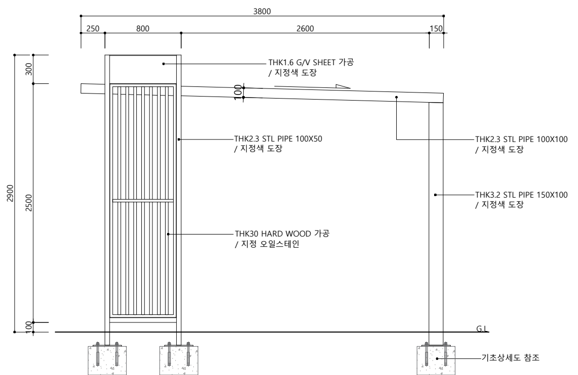
2 입면도 SCALE(A3): 1/40
