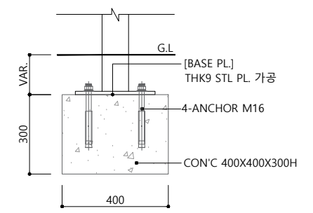
4 기초상세도 SCALE(A3): 1/20
