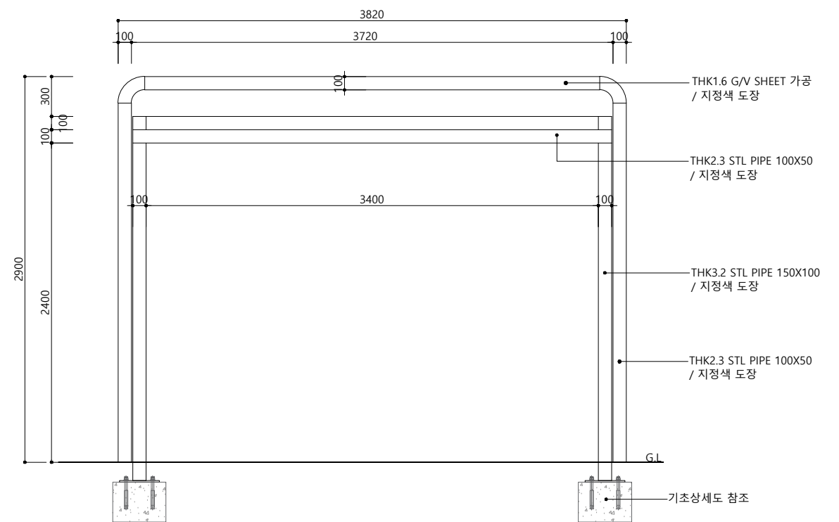
3 측면도 SCALE(A3): 1/40
