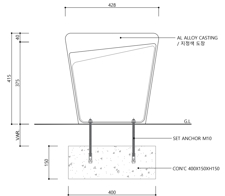
3 측면도 SCALE=A3 : 1/10
